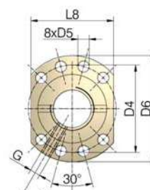
Schema di foratura 2 secondo DIN 69051
