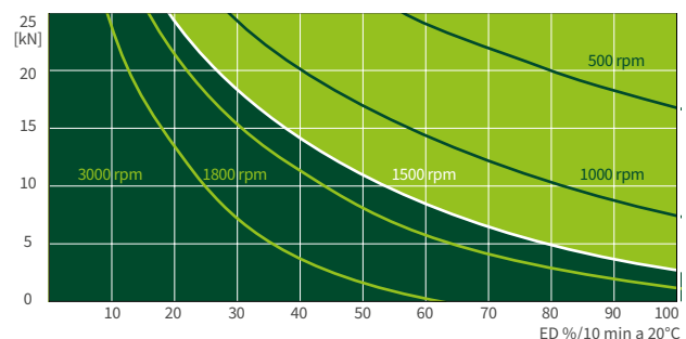
Rapporto „L“ (24:1)
